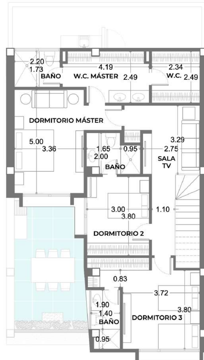
PLANTA ALTA Área: 113.12 m 2
