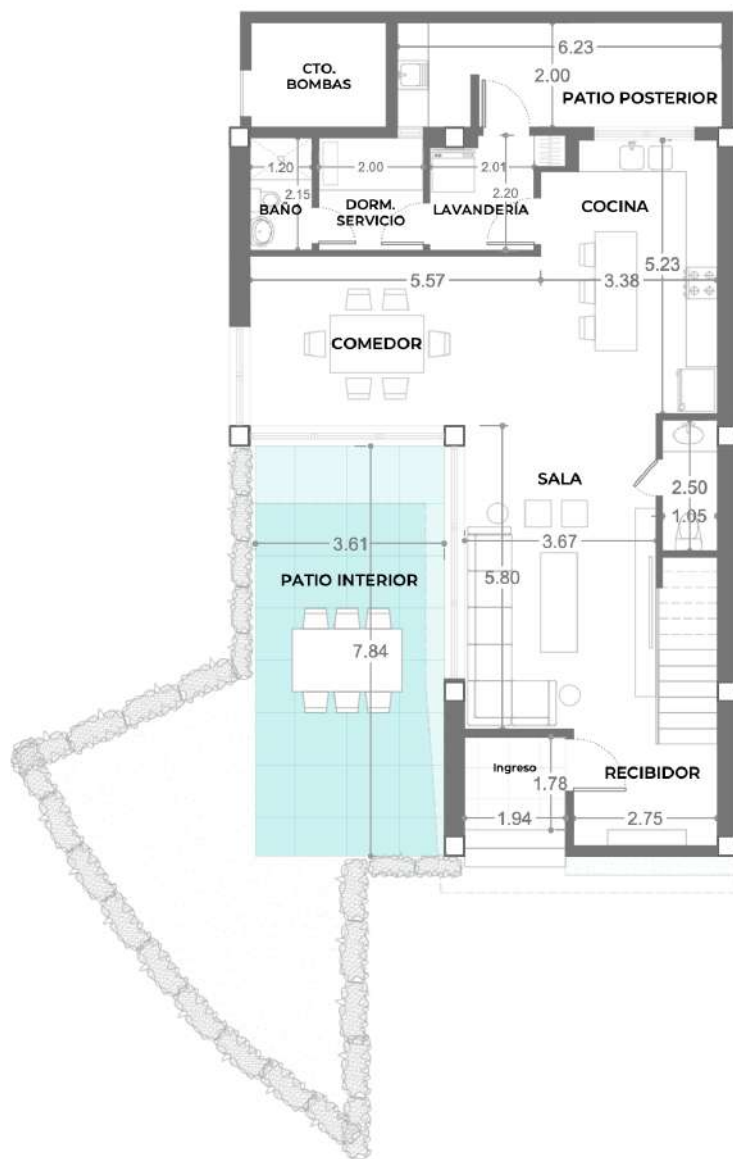
PLANTA BAJA Área: 100.73 m 2
