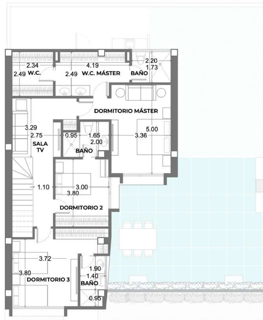
PLANTA ALTA Área: 114.72 m 2
