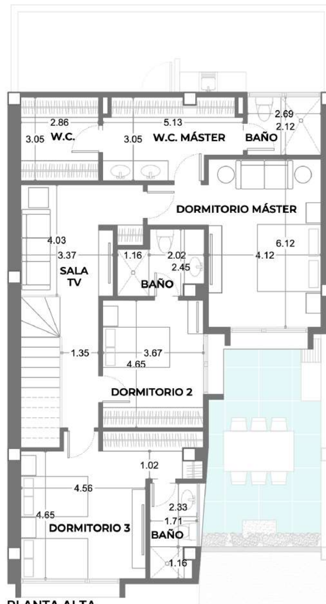
PLANTA ALTA Área: 112.01 m 2
