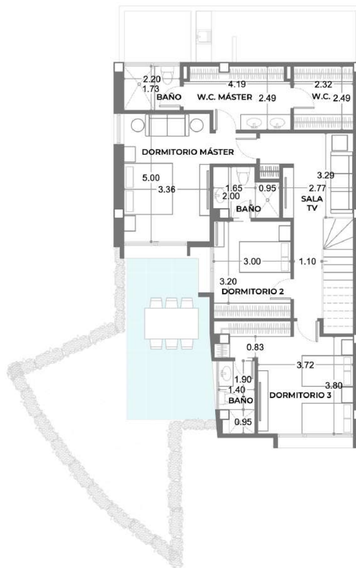
PLANTA ALTA Área: 114.70 m 2
