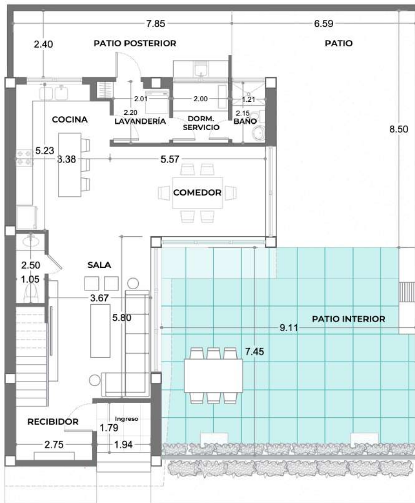
PLANTA BAJA Área: 100.70 m 2
