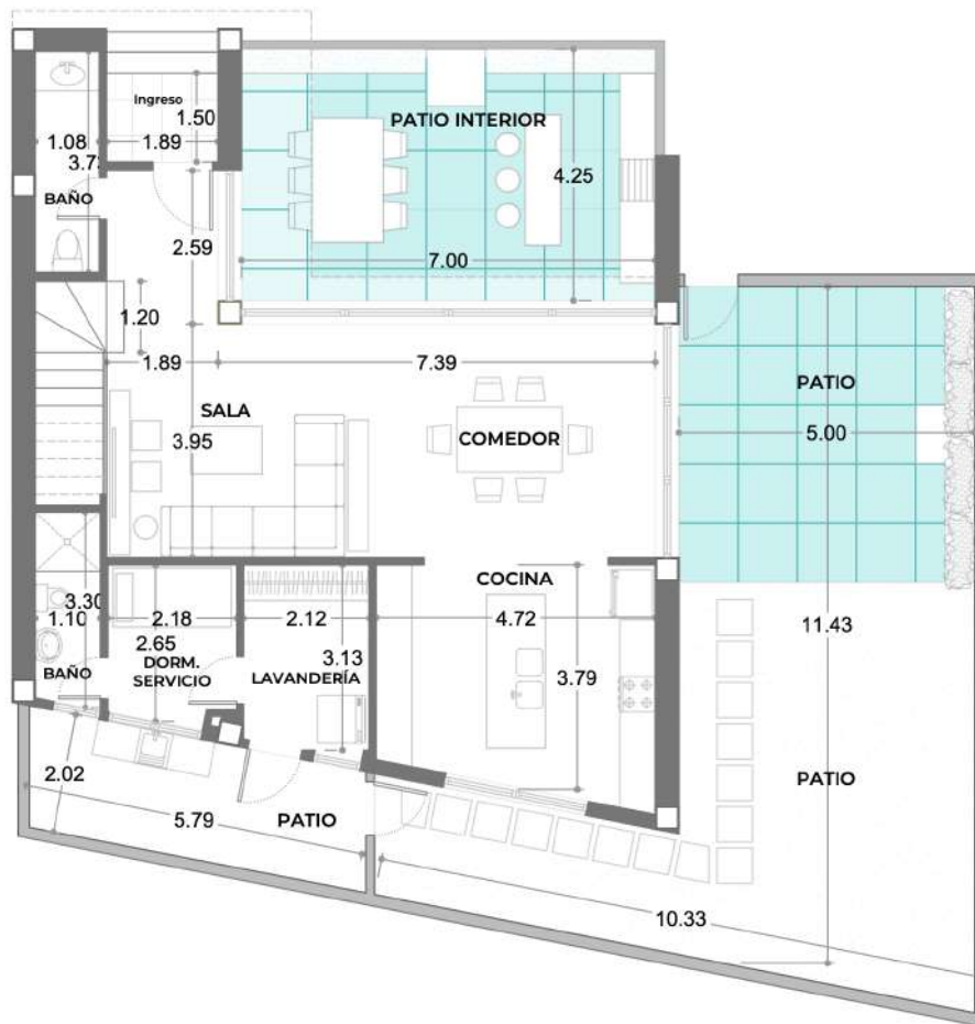
PLANTA BAJA Área: 104.60 m 2
